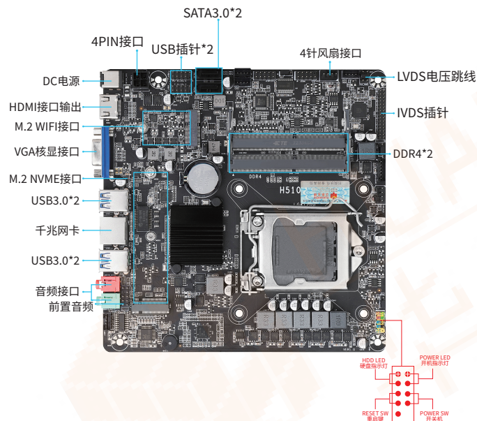
图1-1 H510M-I 主板图解
