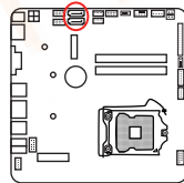
图2-8 SATA接口
